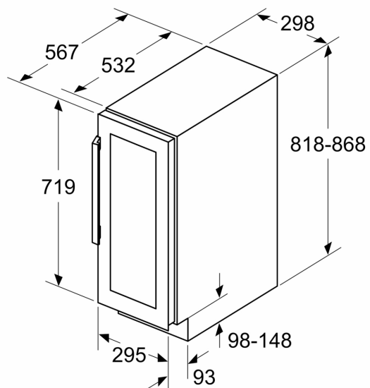
Wymiary w mm
