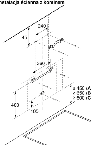
Wymiary w mm Instalacja ścienna z kominem
