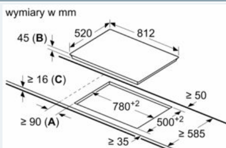
Rysunki wymiarowe
