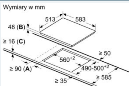
Rysunki wymiarowe
