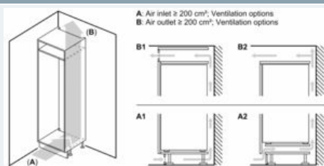
Rysunki wymiarowe
