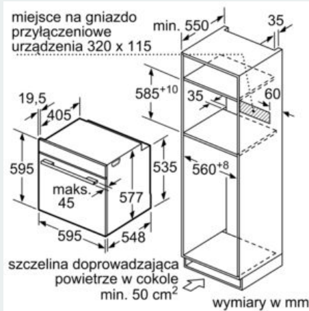
Rysunki wymiarowe
