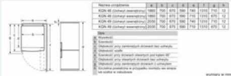
Rysunki wymiarowe
